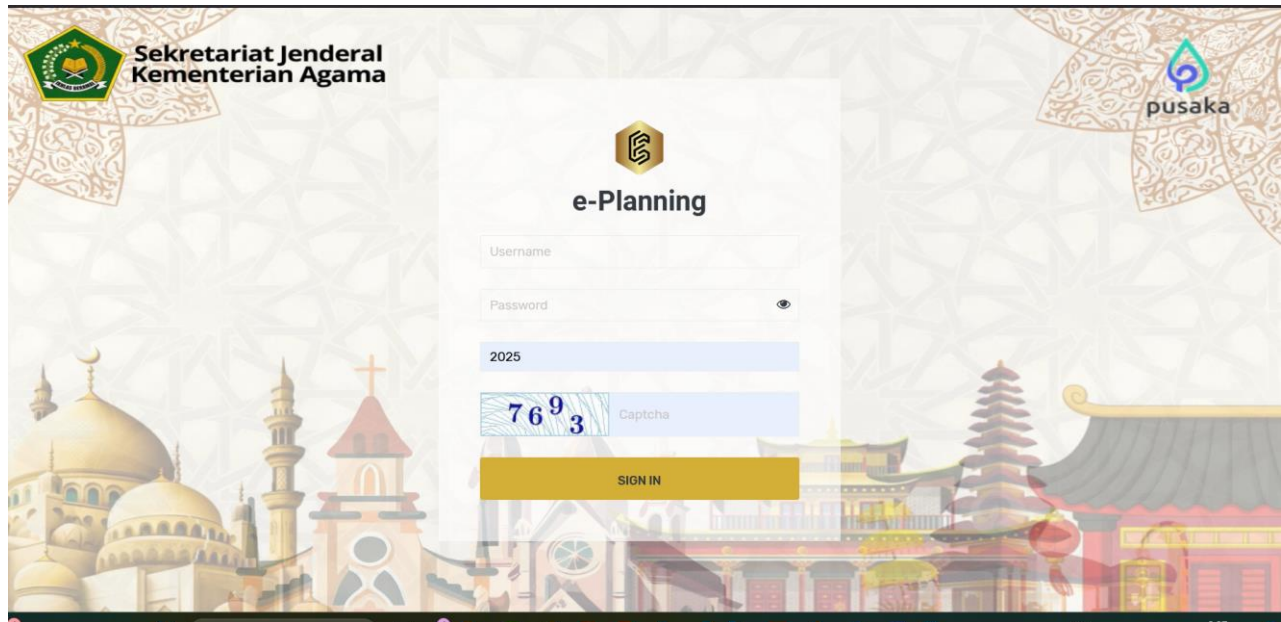
Gambar 59 Jendela Login
