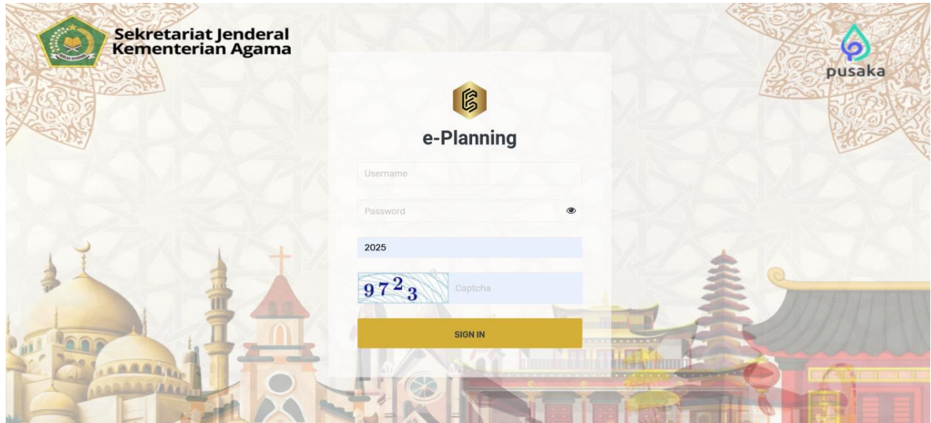
Gambar 1 Login
