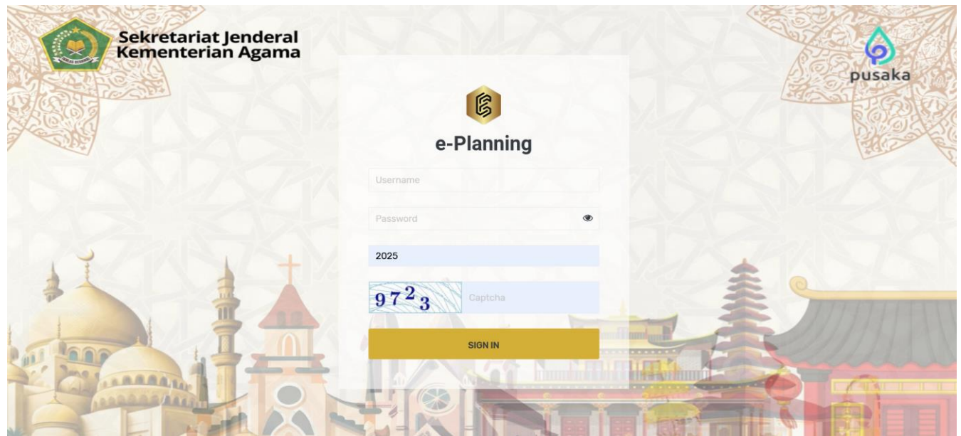
Gambar 2 Jendela Login
