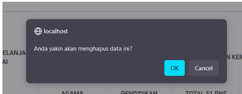
Gambar 66 Hapus Usulan
